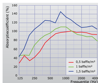
Geluidsabsorptiewaarden bij een baffle van 1200 x 600 x 50 mm
